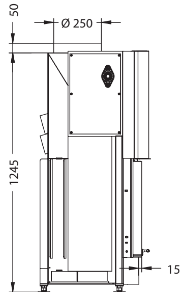
Seitenansicht M~1:20
